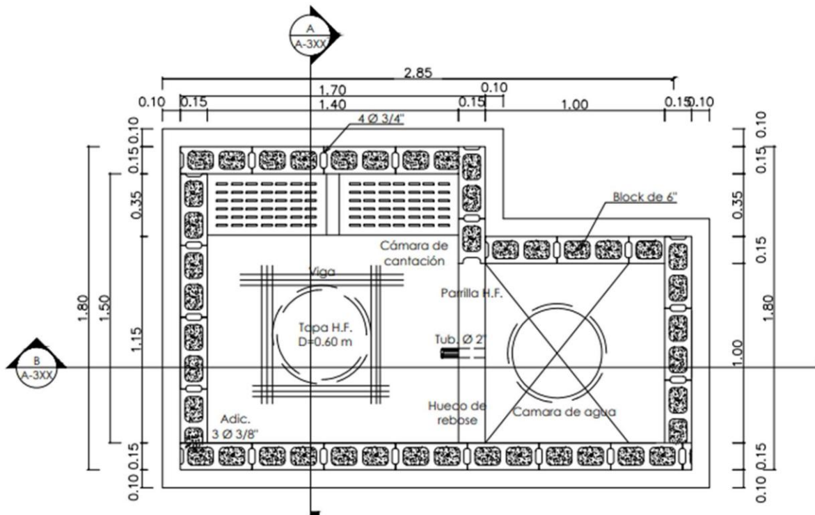
Imbornal de una (1) parrilla
